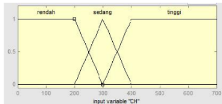
Gambar 8 Variabel Curah Hujan
