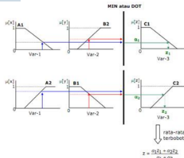
Gambar 6 Inferensi dengan menggunakan Metode Tsukamoto
