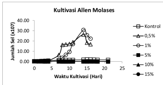
Gambar 2. Kurva Pertumbuhan
