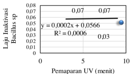
Gambar 6. Laju Inaktivasi bakteri Bacillus sp susu pasterisasi metode termal UV dan ozon
