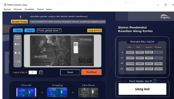
Gambar 10. Tampilan Menu Pendeteksi Keaslian Uang
