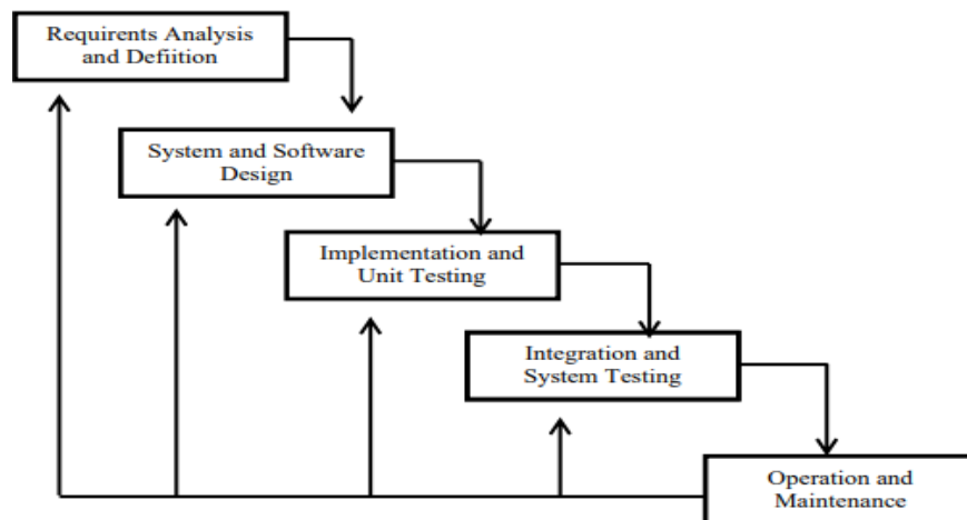
Gambar 1. 2 Metode Waterfall Menurut Ian Sommerville (Submber: Irawati dan Darwati, 2020).
