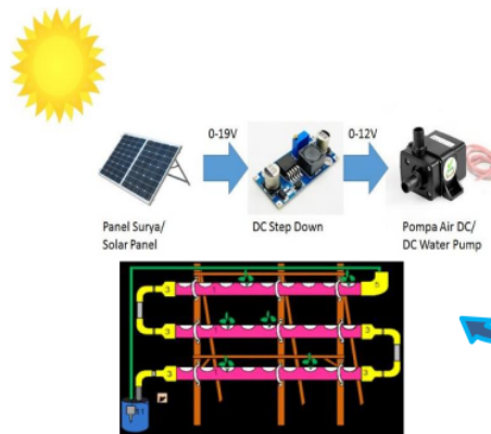
Gambar 3. Metode DFT pada Hidroponik yang dikombinasi dengan Otomatisasi dan Tenaga Surya
