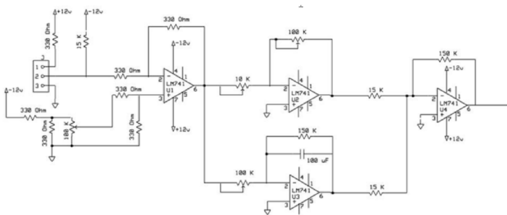
Gambar 2. Desain rangkaian PI analog
