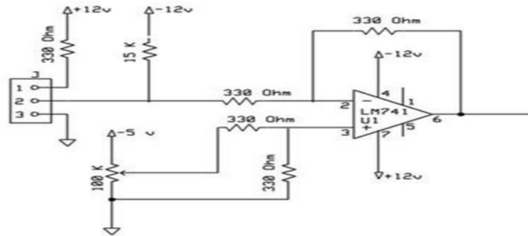
Gambar 3. Rangkaian Error Detector
