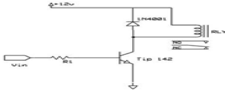
Gambar 5. Perencanaan Rangkaian Driver Katup Solenoid
