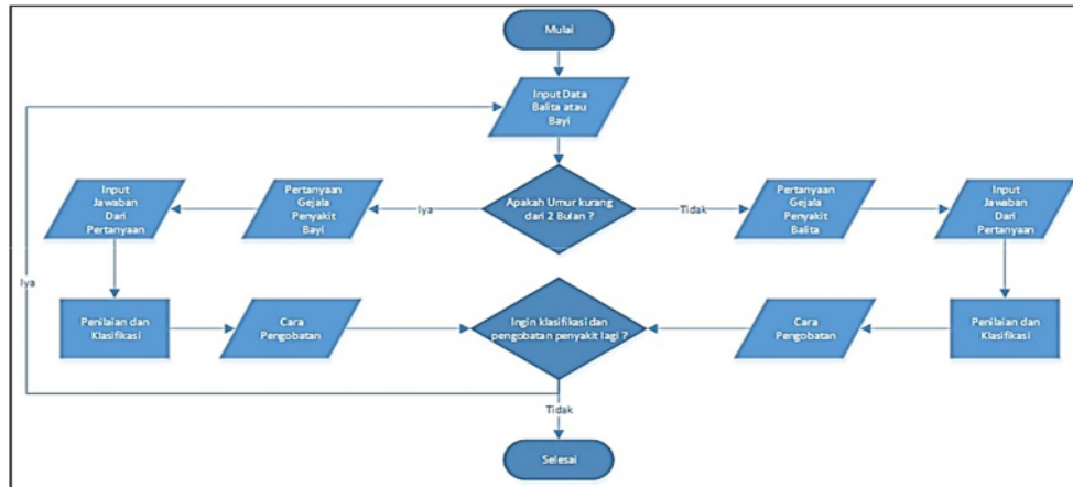
Gambar 2. System flowchart aplikasi imci berbasis android
