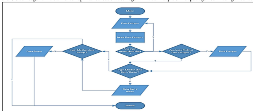
Gambar 3. System flowchart aplikasi berbasis web
