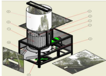
Gambar 4. Alat Peniris (Sumber [7])
