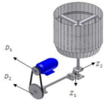
Gambar 3. Sistem transmisi
