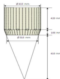
Gambar 2. Desain tabung pengatus
