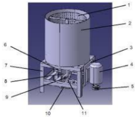
Gambar 1. Gambar mesin peniris/spinner [6]
