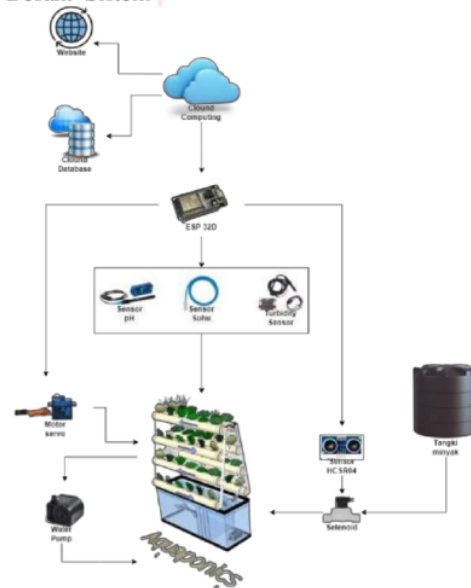
Gambar 9. Desain Sistem
