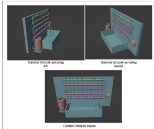
Gambar 11. Desain 3D
