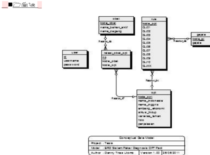
Gambar 9. ERD pada Sistem Pakar Diagnosis OPT Padi Sawah
