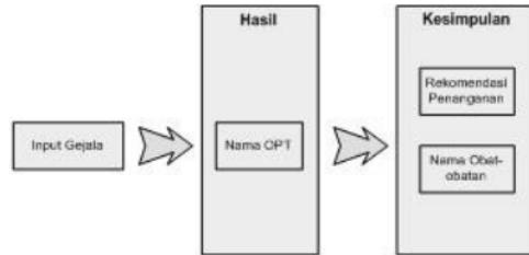
Gambar 5. Penerapan Inferensi Runut Maju ( forward chaining ) pada Sistem Pakar Diagnosis OPT Padi
