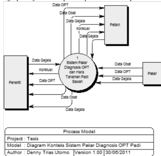
Gambar 7. Diagram Konteks Sistem Pakar
