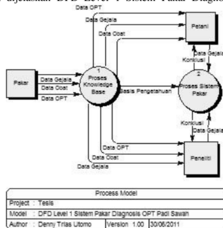
Gambar 8. DFD Level 1 Sistem Pakar
