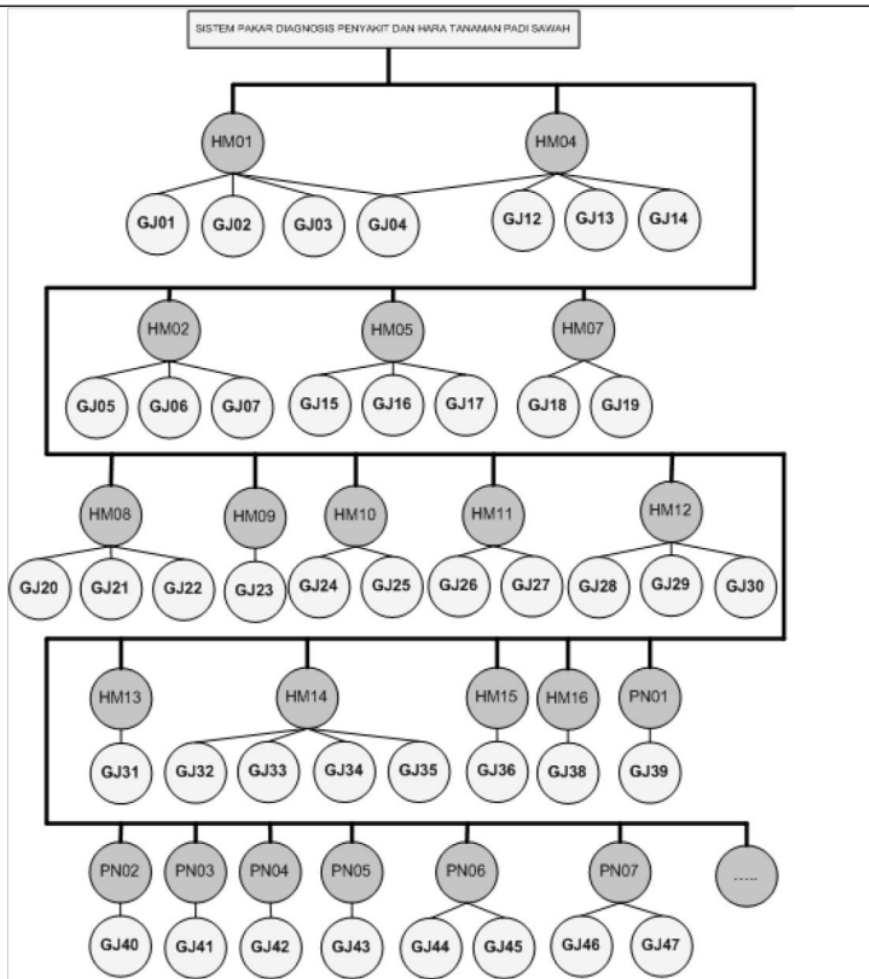
Gambar 3. Knowledge Representation Tree pada OPT Tanaman Padi
