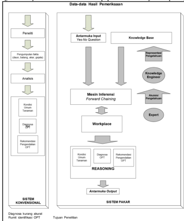
Gambar 1. Konsep pemikiran (Sistem Pakar Diagnosis OPT)
