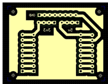
Figure 5. Design of Wemos D1 Mini PCB Shield
